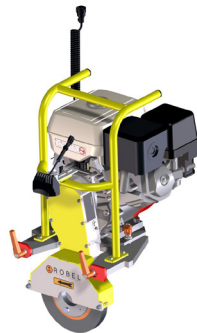
Grinding disc module GX 270
